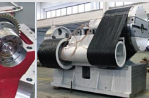
testa porta pezzo per rettifiche cilindro laminazione head holding the workpiece for the rolling cylinder rectifications
