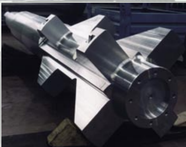
albero per mandrino avvolgitore Coil spindle tree to Coil
